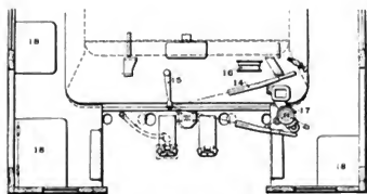
Fig. 2959. Plan.
